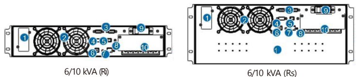
6/10 kVA (R)
